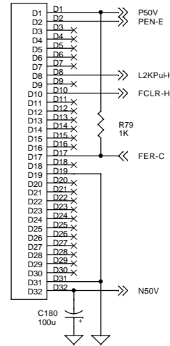
XP11D ERNI-41612-E160
