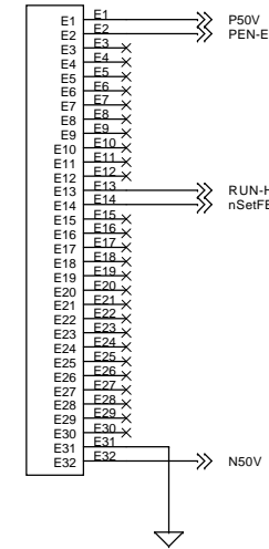
XP11E ERNI-41612-E160
