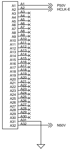
XP11A ERNI-41612-E160
