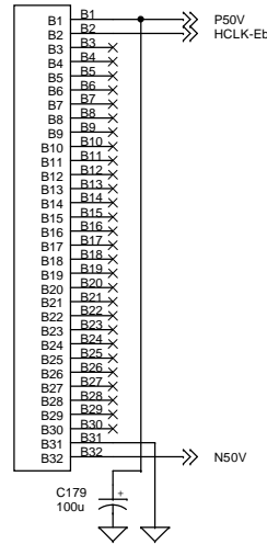
XP11B ERNI-41612-E160
