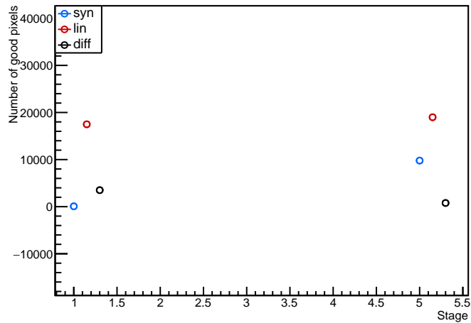
Module: Ox11, A11_Chip4 (FE4) discbumpscan Evolution plot (98<occupancy<102)
