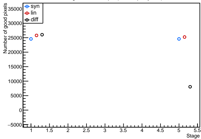
Module: Ox11, A11_Chip4 (FE4) analogscan Evolution plot (97<occupancy<103)
