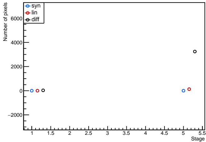
Module: Ox11, A11_Chip4 (FE4) analogscan Evolution plot (0<occupancy<98)
