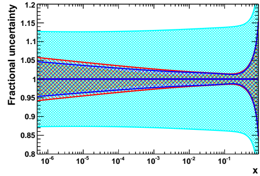
(d) Strange quark distribution.
